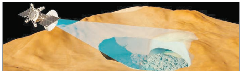
Un estudio con datos de radar detectó un tubo de lava vacío bajo Venus
