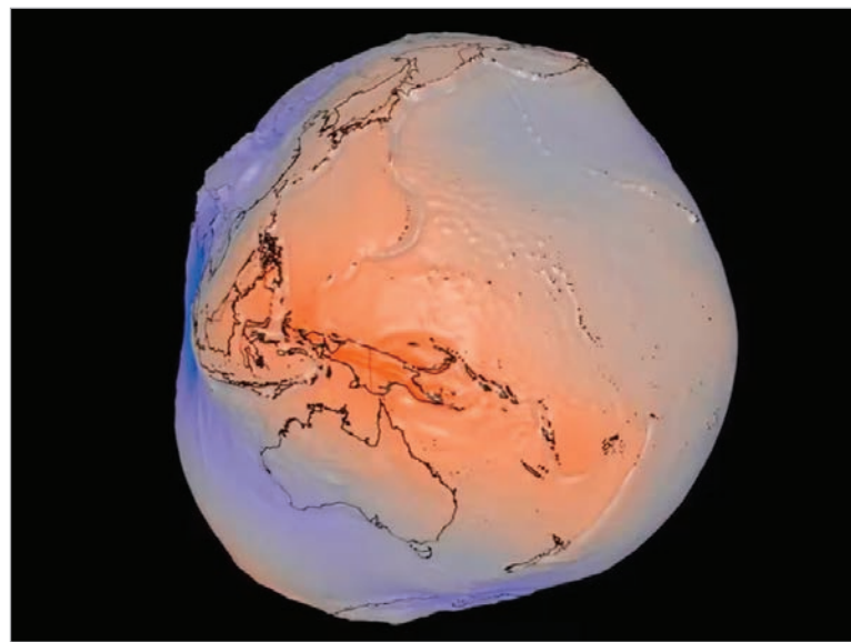
La visualización revela que la Tierra no es una esfera perfecta, sino un cuerpo con variaciones determinadas por su gravedad
